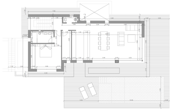
PLANTA BAJA
